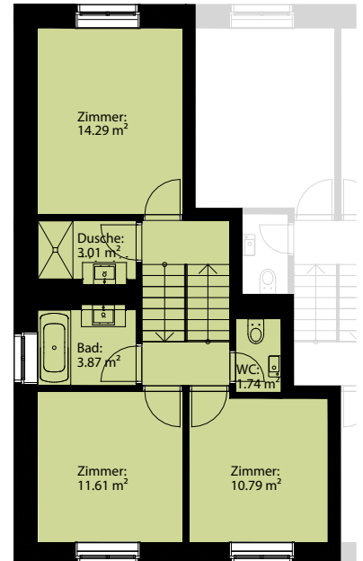
2. Obergeschoss
